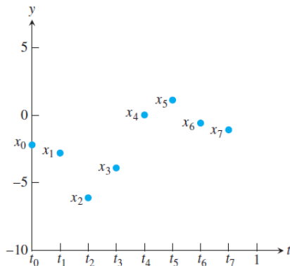
Figura 4: Componentele lui x privite ca o serie de timp. Transformata Fourier este o modalitate de a calcula polinomul trigonometric care interpoalează aceste date.
